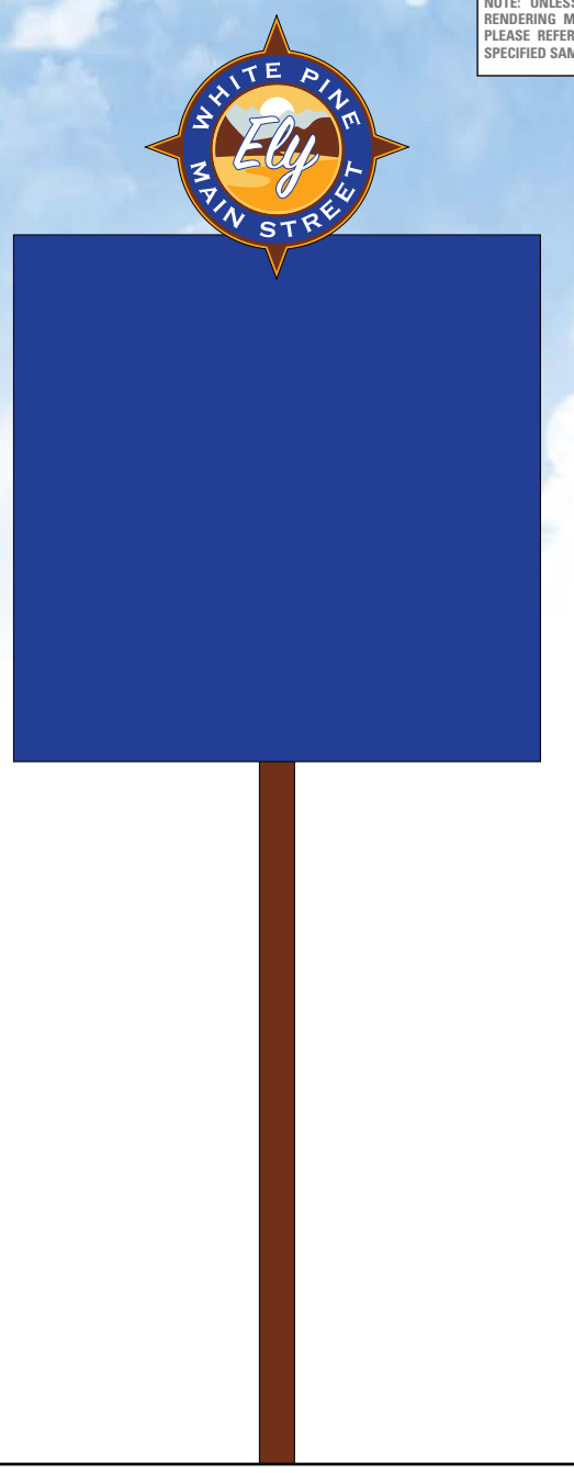
DRAWING 3 SIGN TYPE D1 BACK VIEW SCALE: 1/2" = 1'-0"
